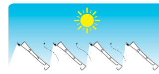
Protection solaire maximale et ventilation naturelle.
